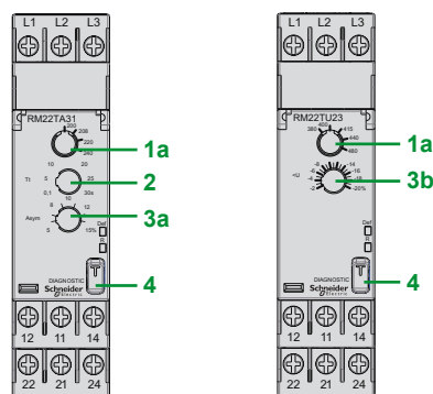
RM22TA
