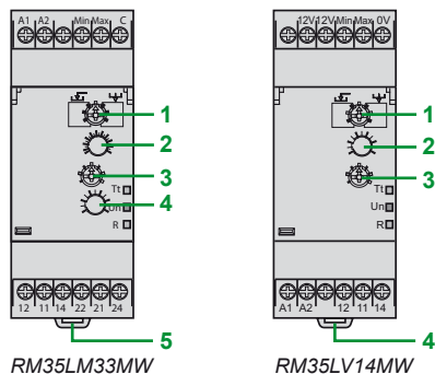
RM35LM33MW
